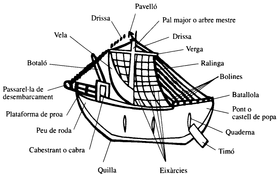
FIG. 5. Representació esquemàtica de la navis oneraria que apareix als anversos dels asos de la primera emissió d' Ilercavonia-Dertosa .
