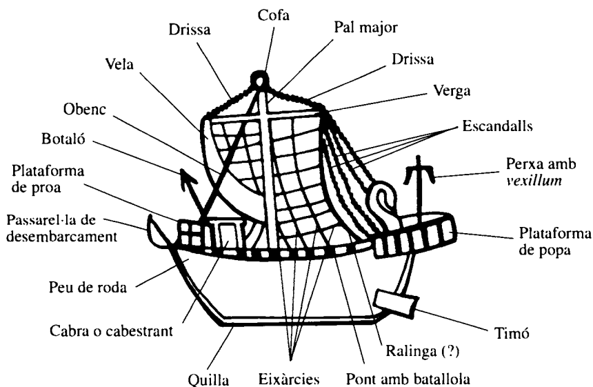
FIG. 11. Representació esquemàtica de la navis oneraria del revers dels asos de la segona emissió d'Ilercavonia-Dertosa.
